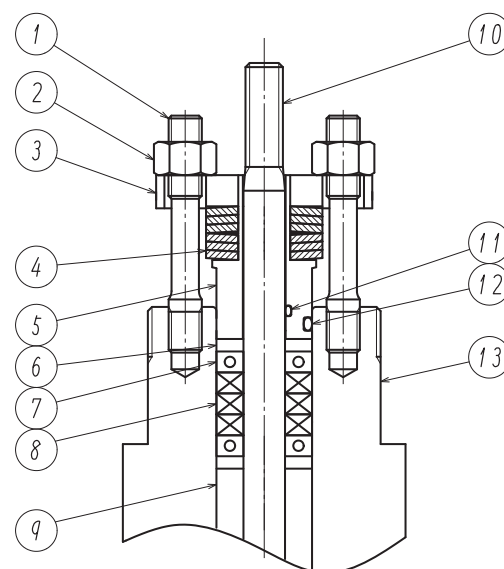
图 10-2 低泄露密封填料系统结构图 (膨胀石墨规格)
