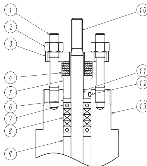
图 10-1低泄露密封填料系统结构图 (聚四氟乙烯编织物规格)
