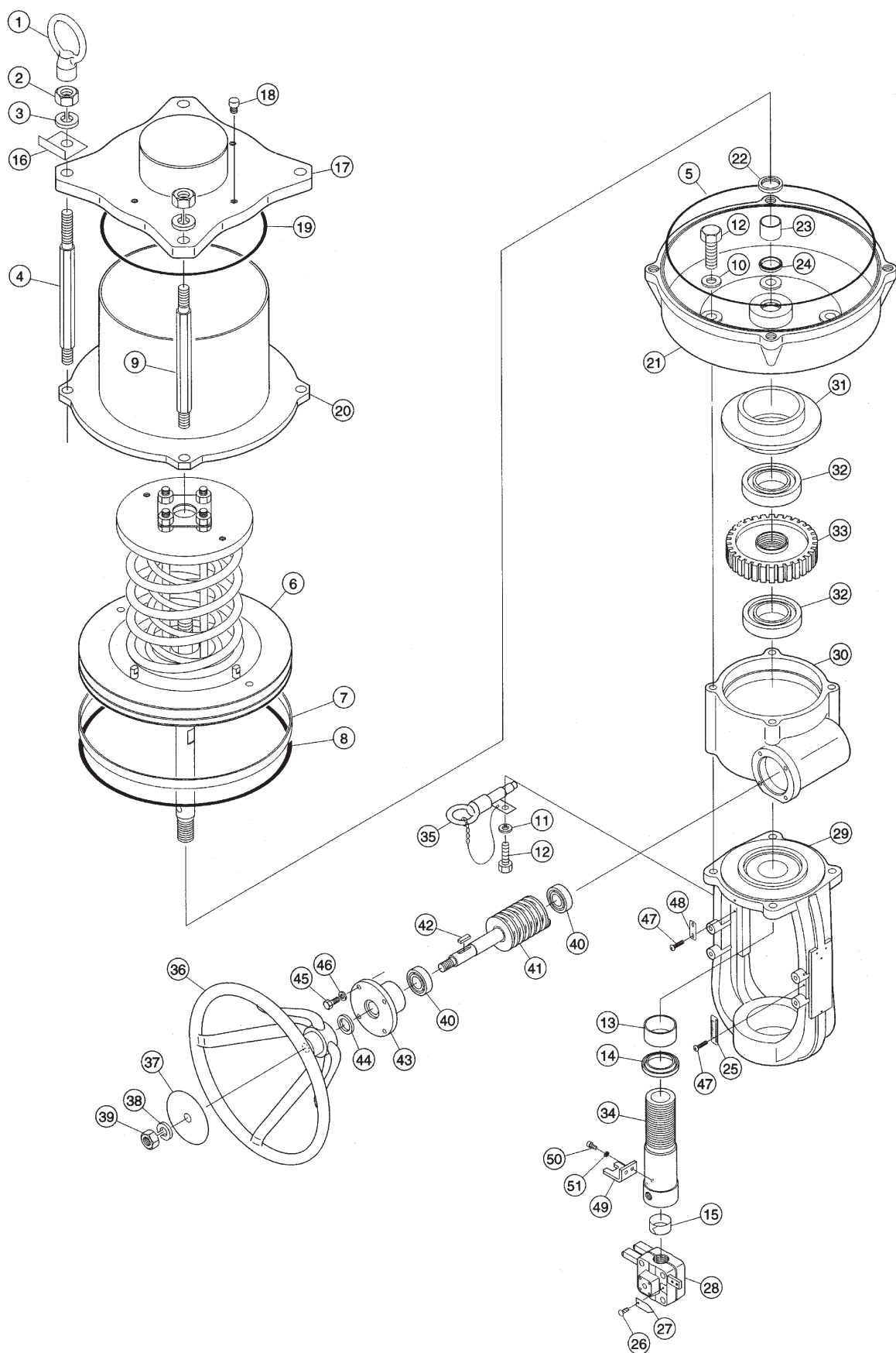
图 4-22 型号 PSA6R
