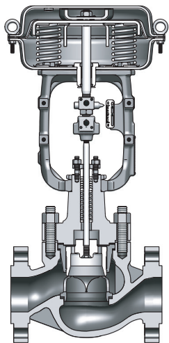
图 1-1 压力平衡笼式调节阀型号 HCB
