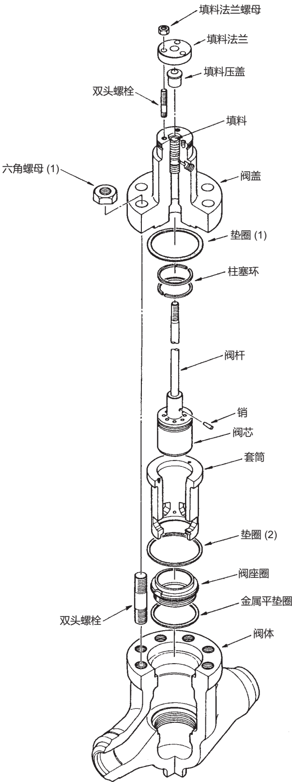
图 4-2 型号 HPC 调节阀
